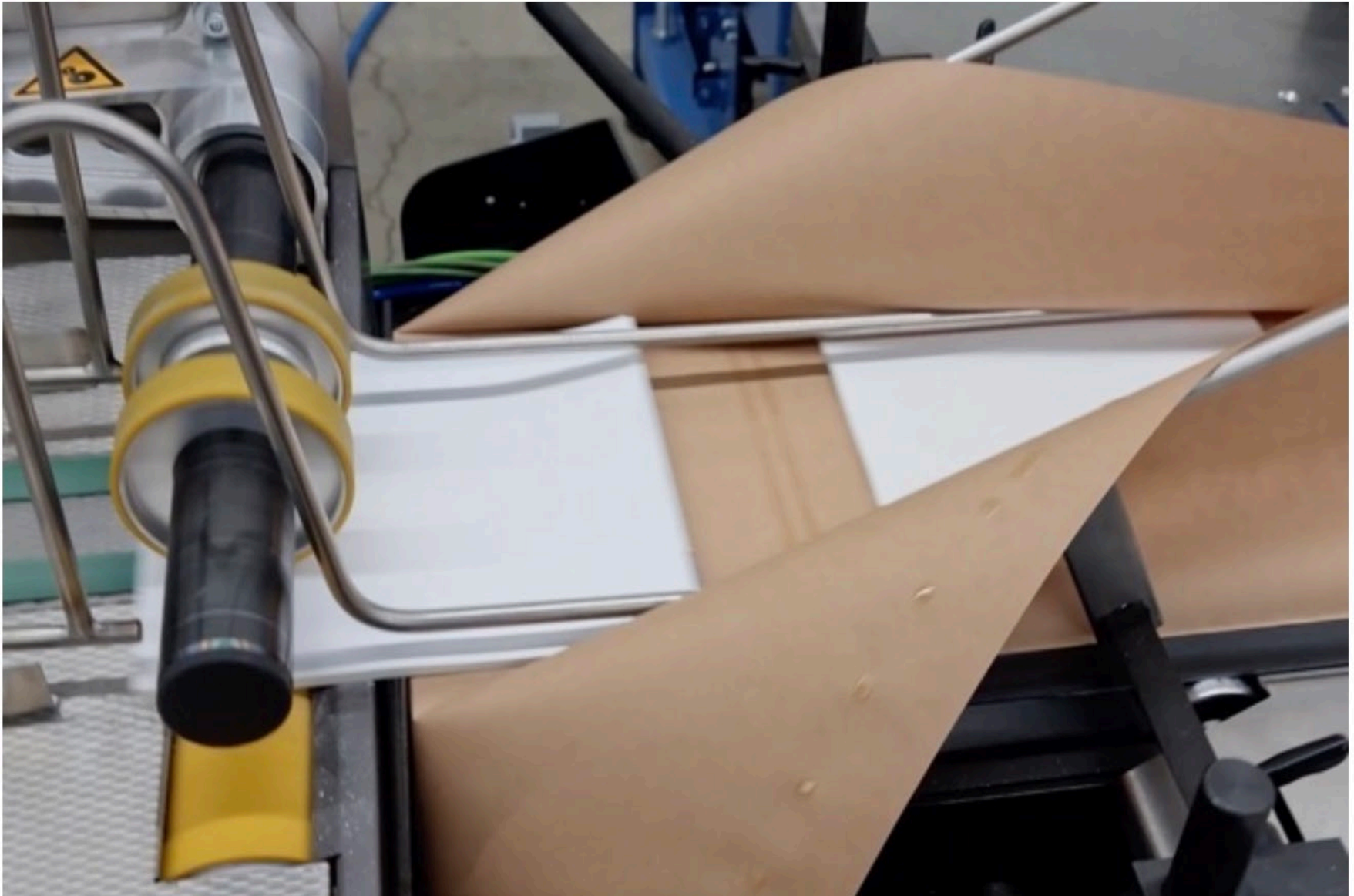
Buhrs-Papierverpackungssystem für 100 % geprüfte Verpackung
